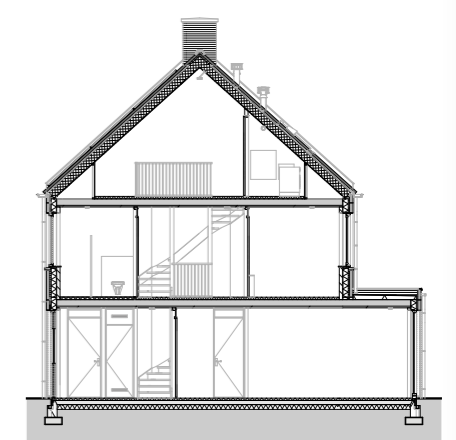
Doorsnede
